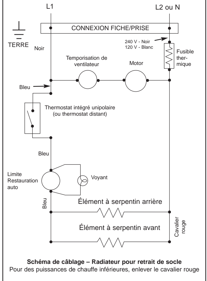
Fig. 3 Câblage avec thermostat monté dans le radiateur
