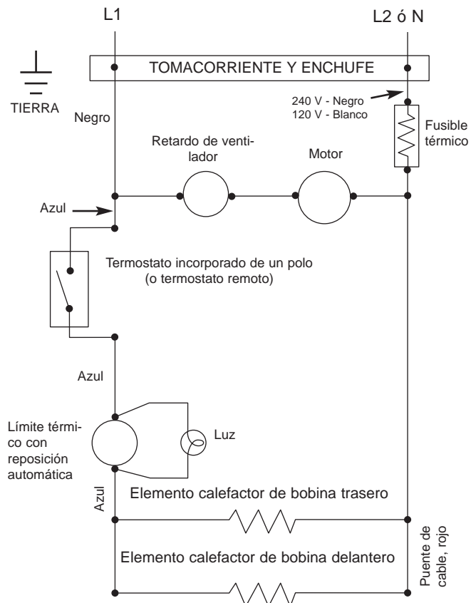
Diagrama de conexionado – Calefactor a ras del piso Para funcionamiento de baja potencia retire el puente de cable rojo
